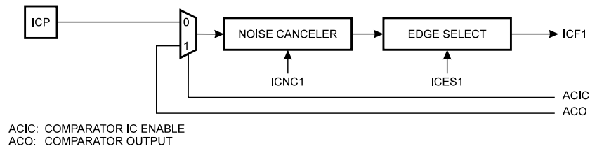
图 31 ICP 引脚原理图
