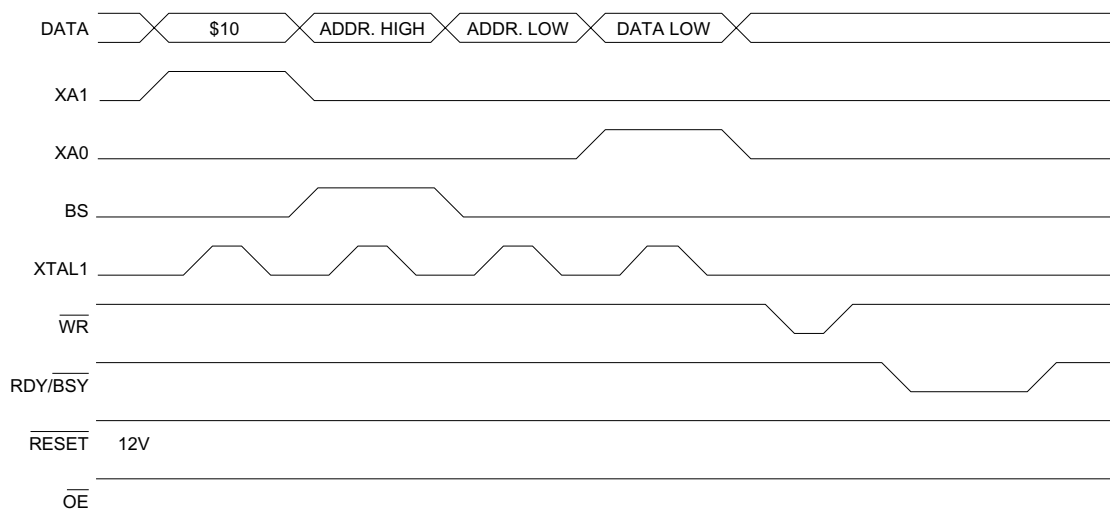
图 50 编程波形一
