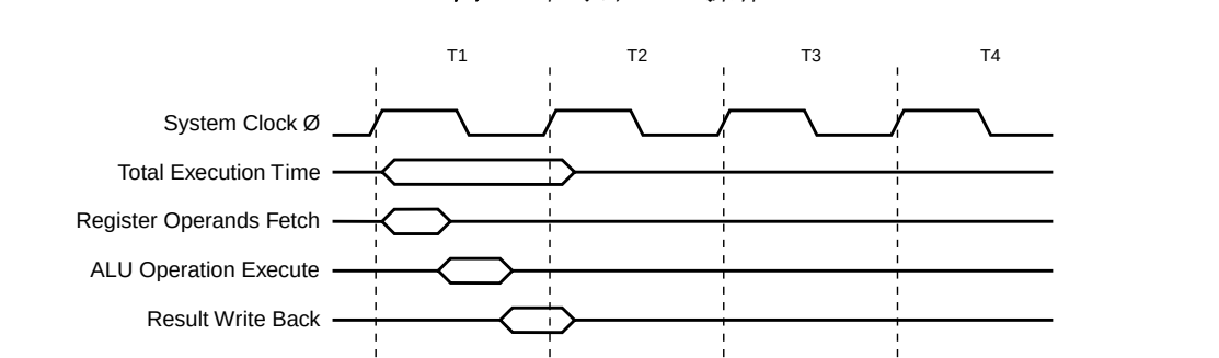
图 21 单时钟 ALU 操作
