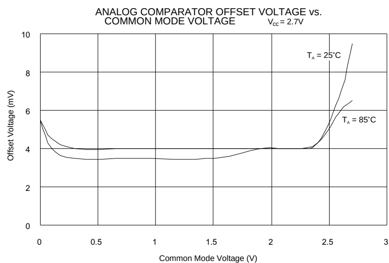
图 65 模拟比较器偏置电压与共模电压的关系
