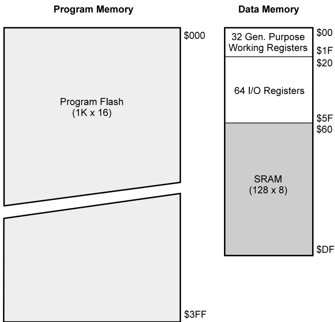
图 5 内存映像
