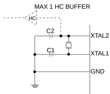
图 2 振荡器连接
