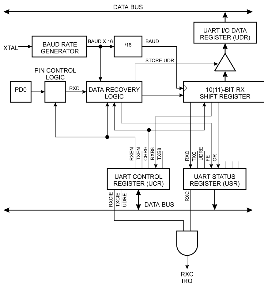
图 35 UART 接收器
