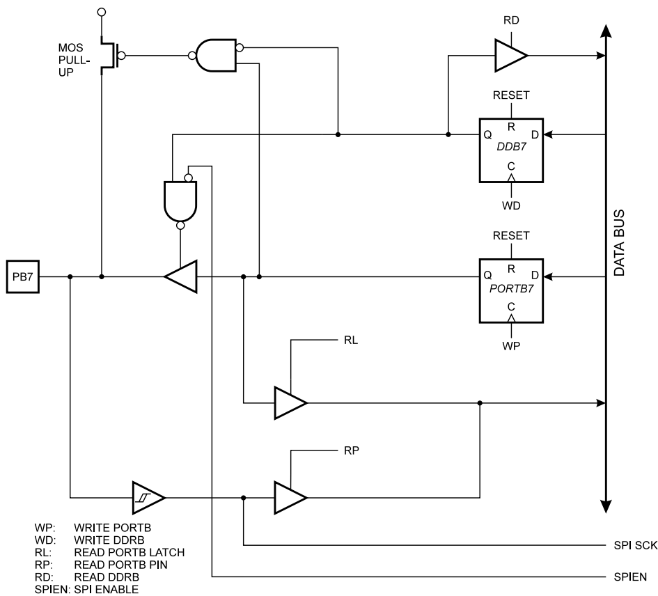
图 43 B 口示意图 (PB7)
