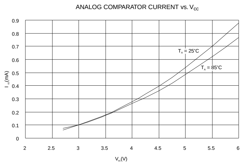
图 63 模拟比较器电流与电压的关系
