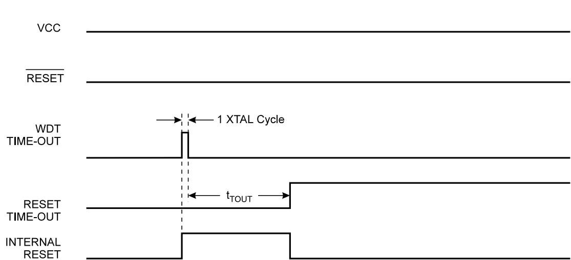
图 27 工作期间的看门狗复位
