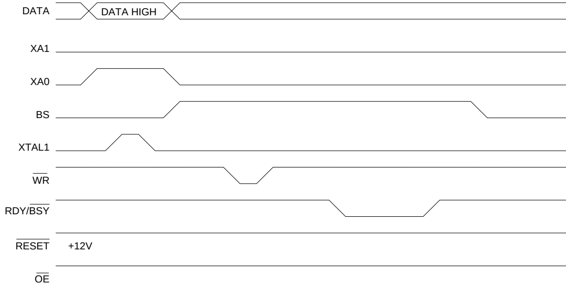
图 51 编程波形二
