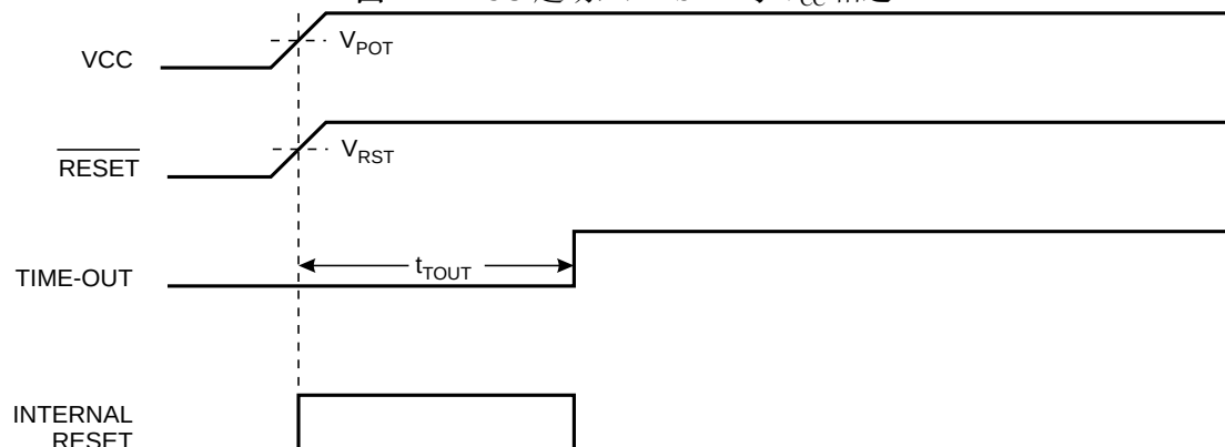
图 24 MCU 起动，/RESET 与 V_{CC} 相连
