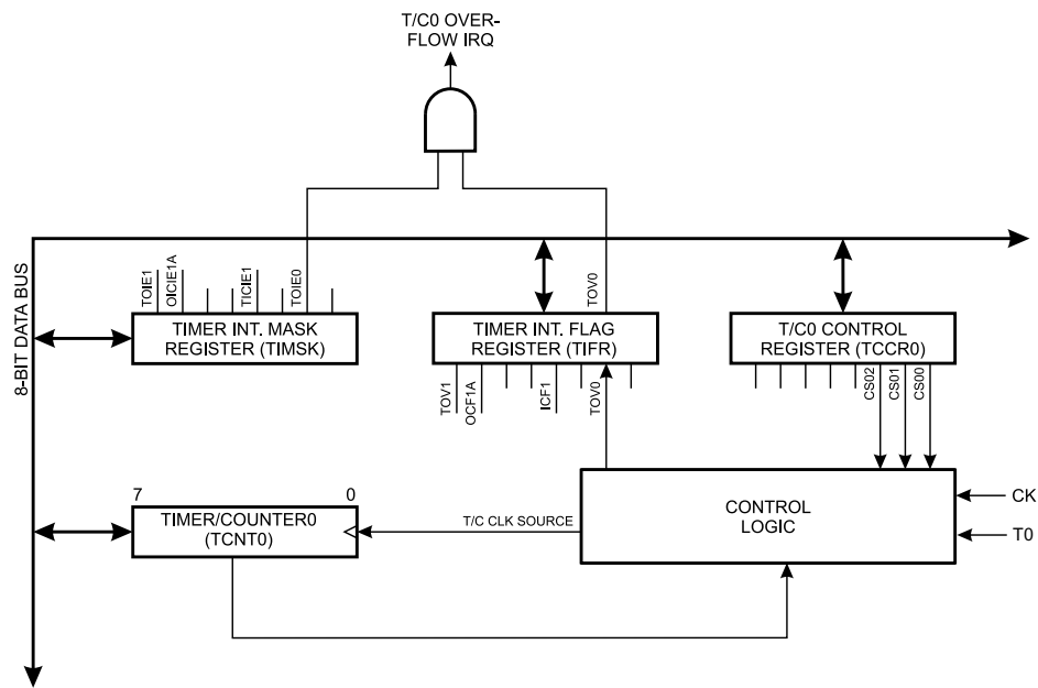
图 29 T/C0 工作框图
