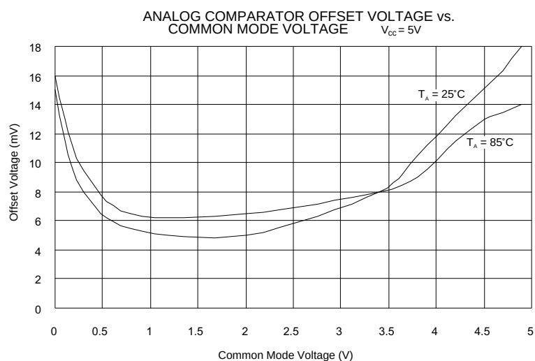
图 64 模拟比较器偏置电压与共模电压的关系
